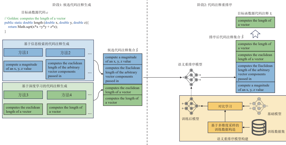
图 2 SRBCS 工作流程概览
