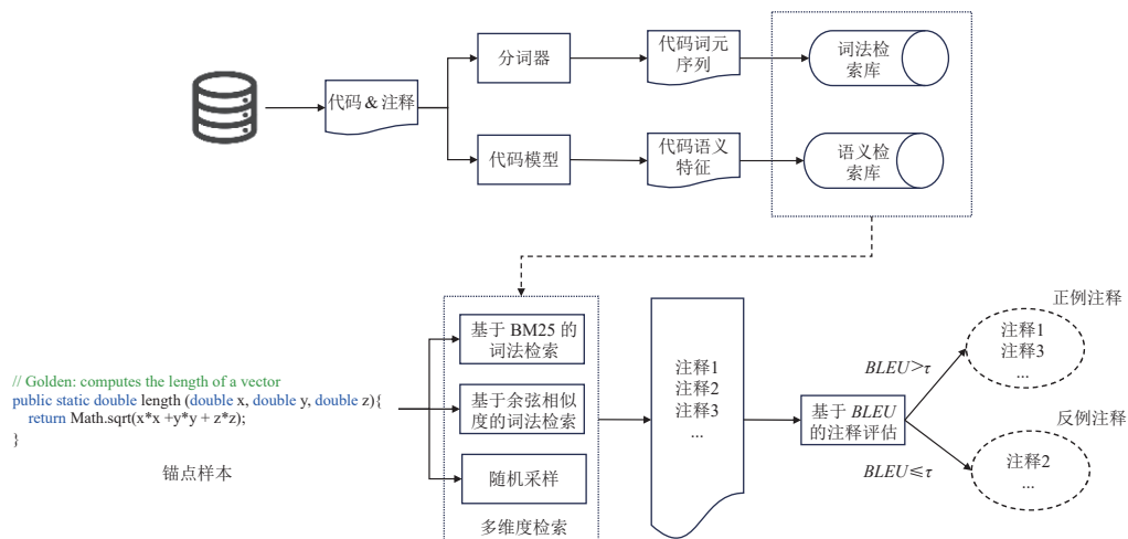
图 3 多维度正负样本对构造流程
