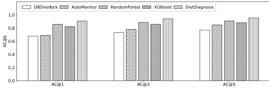
图3 单节点异常诊断场景中各方法 AC@k 对比
