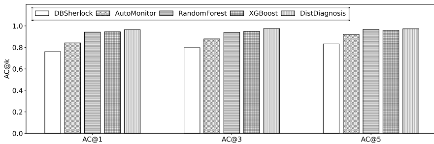
图 4 多节点异常诊断场景中各方法 AC@k 对比
