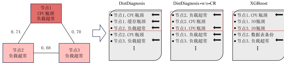
图 9 CPU 瓶颈+负载超常的多节点复合异常时各方法的输出结果
