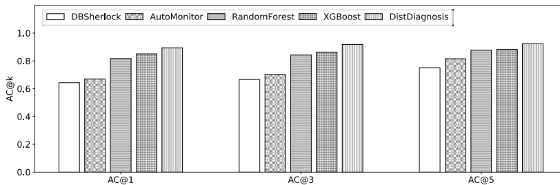
图 6 多节点复合异常场景中各方法 AC@k 对比
