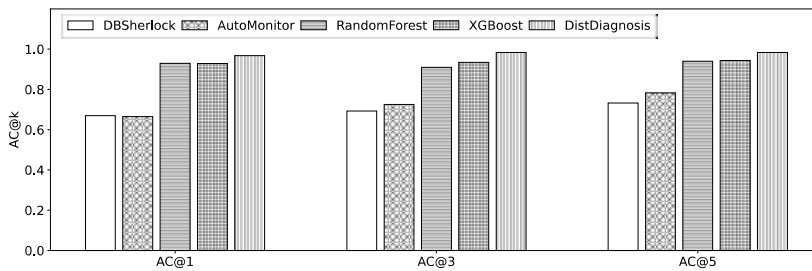
图 5 单节点复合异常场景中各方法 AC@k 对比
