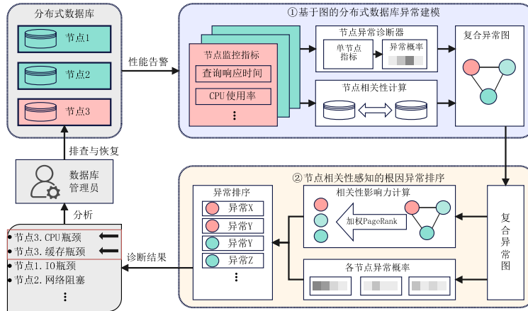
图2 DistDiagnosis方法结构示意图
