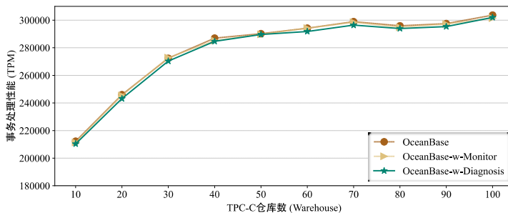
图 7 不同仓库数下 DistDiagnosis 对数据库的性能影响
