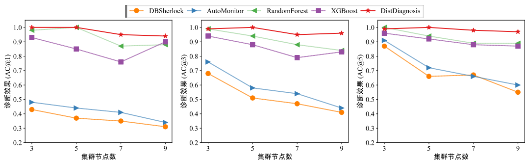
图 8 不同规模集群中的诊断效果对比
