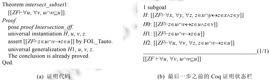
图 1 ZFC 集合论证明器证明环境示例
