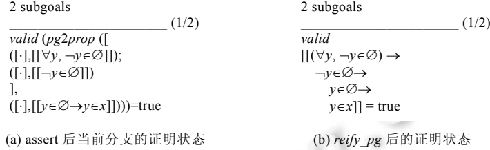
图 5 FOL_Tauto 证明步骤拆解
