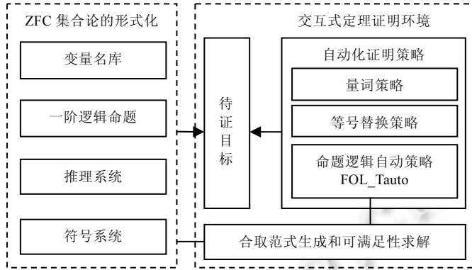
图 2 ZFC 集合论证明器设计框架
