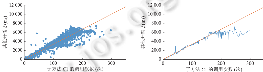
图 9 实例拟合效果图
