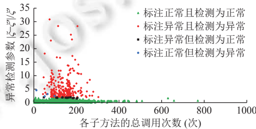
图7 方法重复调用模式实例的检测结果图
