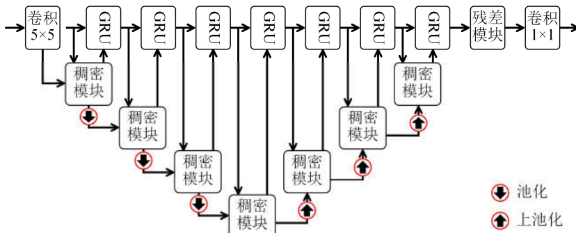
Fig.20 The GRUU-Net architecture for cell segmentation 图 20 用于细胞分割的 GRUU-Net 模型结构
