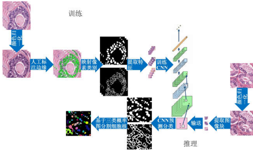
Fig.12 The CNN3 model for nuclear segmentation 图 12 用于细胞核分割的 CNN3 模型
