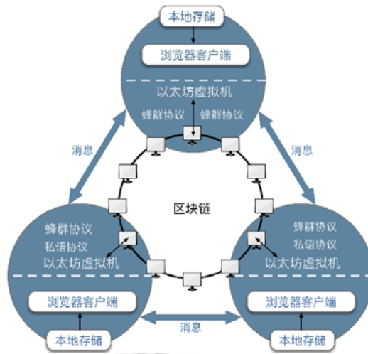
Fig.3 The architecture of Ethereum 图3 以太坊架构图
