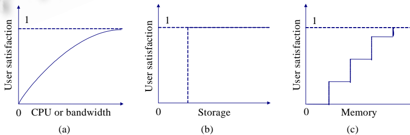
Fig.3 Examples of user satisfaction function 图 3 用户满意函数的例子
