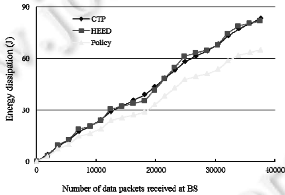
Fig.14 Energy consumption of the WSNs 图 14 任务随机产生场景下,传感器网络的能耗对比
