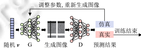
图 6 GANs 的训练过程
