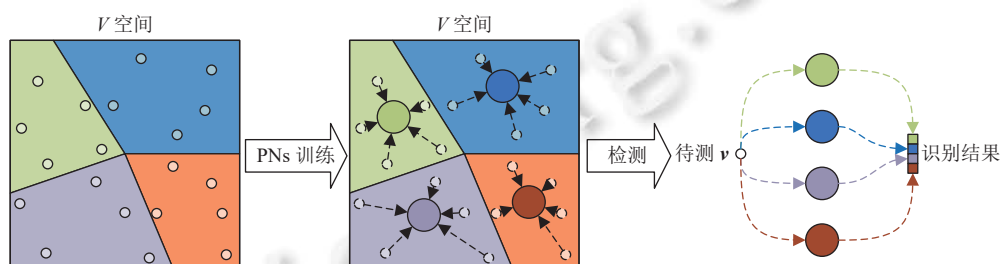
图 18 PNs 的一般流程
