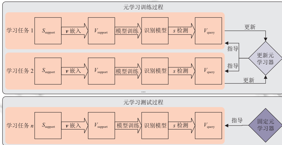
图 11 元学习的一般流程
