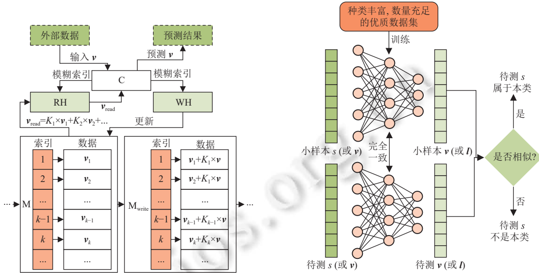
图 16 SNs 的一般流程
