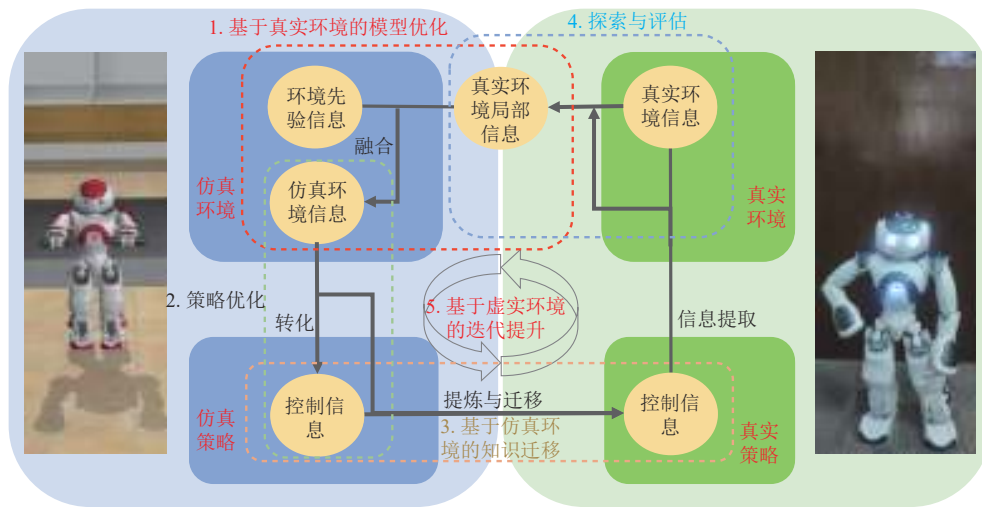
图 1 虚实迁移强化学习流程框架图
