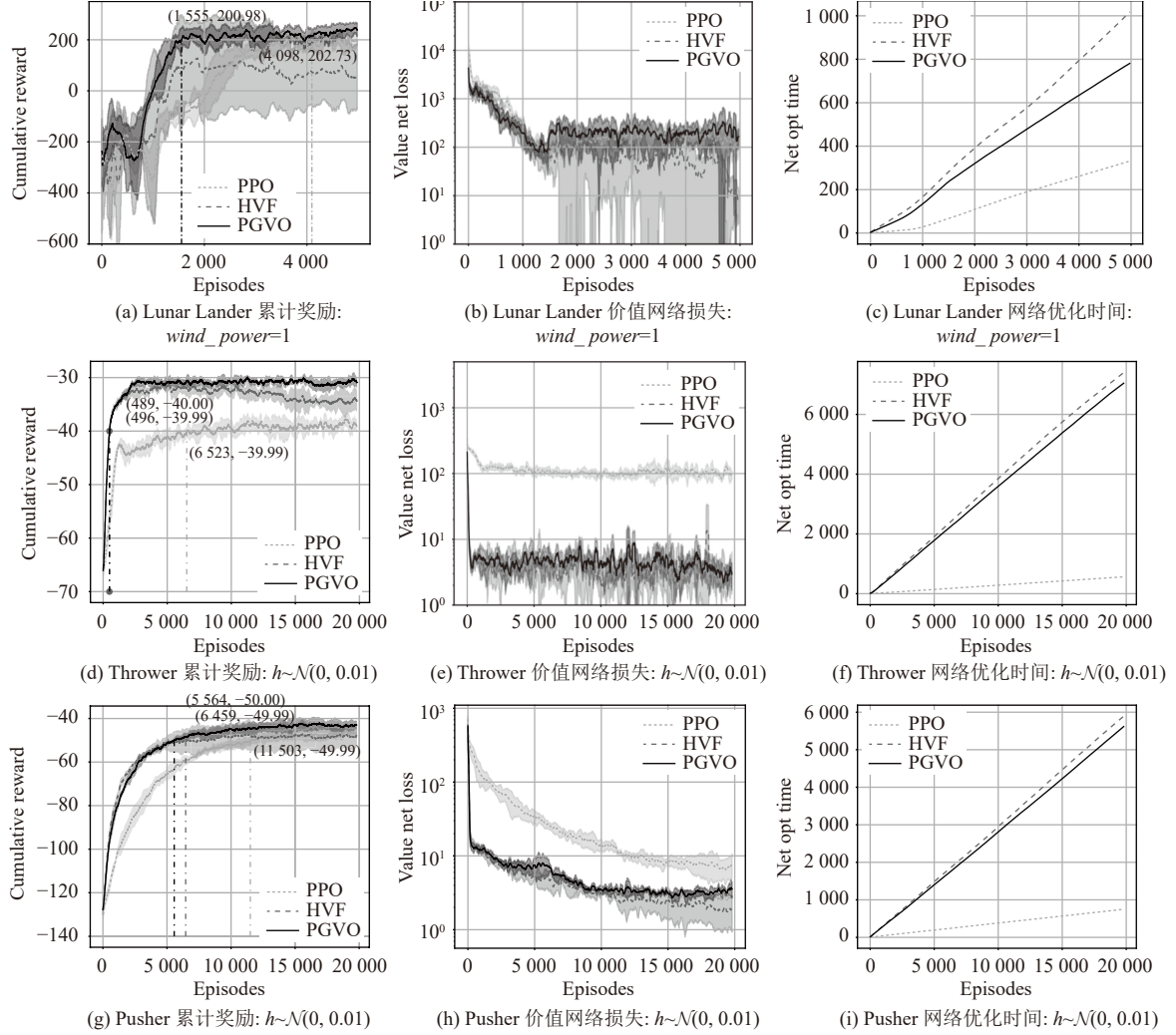
图5 OpenAI Gym 训练过程中累计奖励、网络优化时间和价值损失的可视化曲线
