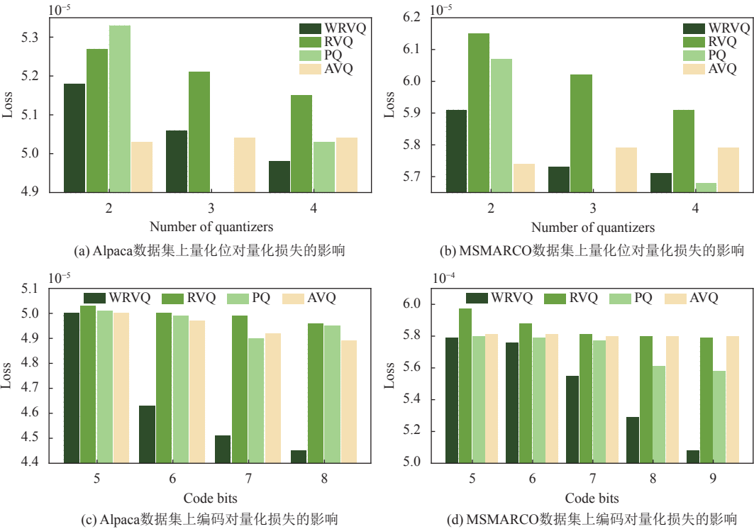
图 5 不同码本大小的抽样训练量化器在两个数据集上的量化损失
