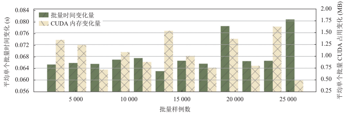
图 7 不同量化向量表征方法在增量索引的时空开销
