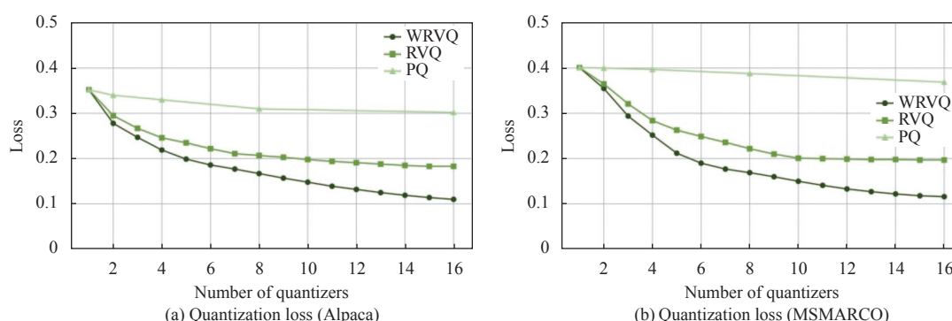
图 4 基于线性残差微调码本的量化器在两个数据集上的量化损失
