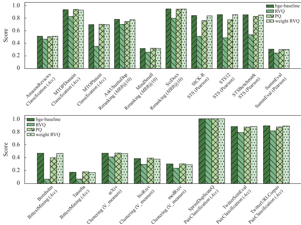
图 6 各量化表征在 MTEB 上的表征能力测试
