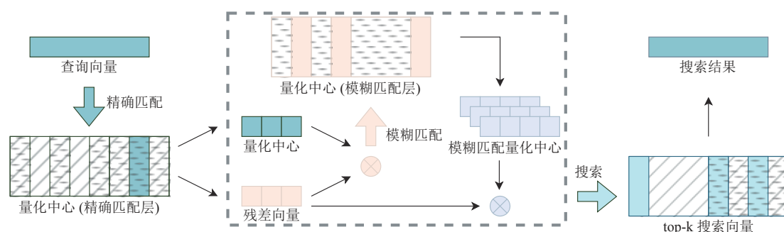
图 3 基于权重向量量化的索引结构
