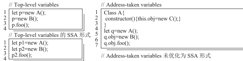
图 8 Panda IR 的 Partial SSA 优化
