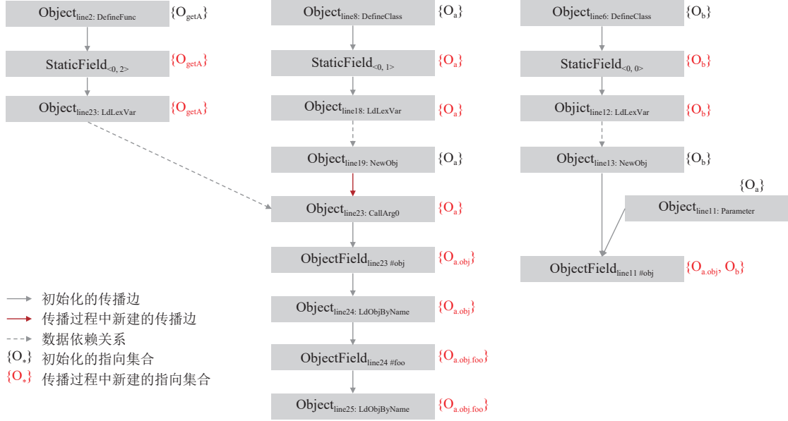
图 5 Panda IR 程序字段敏感性分析的指针流图示例
