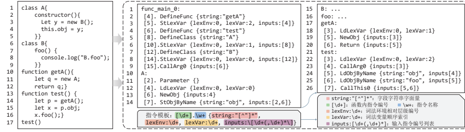
图3 Panda IR 程序中的字段敏感性分析示例
