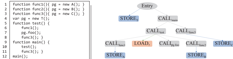
图7 优化数据依赖分析示例
