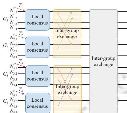
图3 Canopus 共识架构
