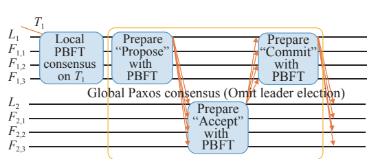
图1 Steward 的 Paxos 复制流程
