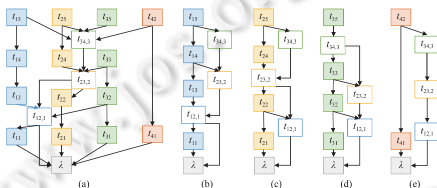
图 13 CAPER 的 DAG 账本结构
