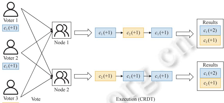
图 10 CRDT 并发控制的执行流程
