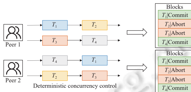
图9 使用确定性并发控制的执行流程
