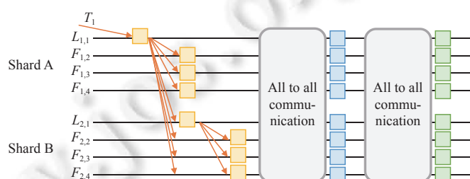
图 12 分布式两阶段提交协议
