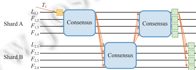
图 11 中心化两阶段提交协议
