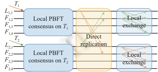
图2 GeoBFT 共识架构
