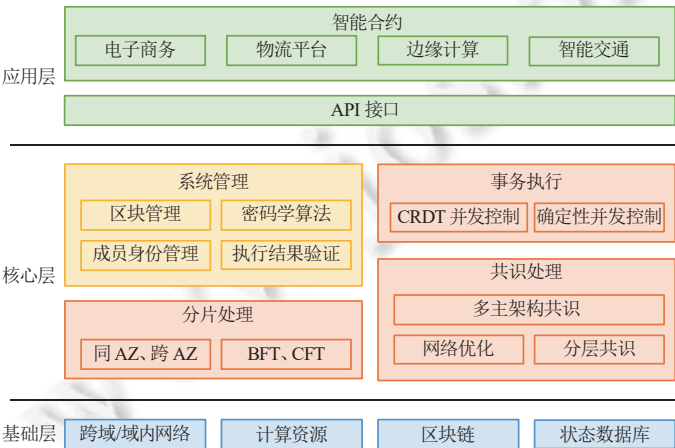
图 14 跨域联盟区块链的层次结构图
