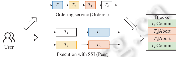
图 8 使用 SSI 并行进行排序和执行阶段
