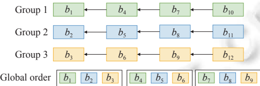
图 5 多主共识算法按轮同步确定全局顺序
