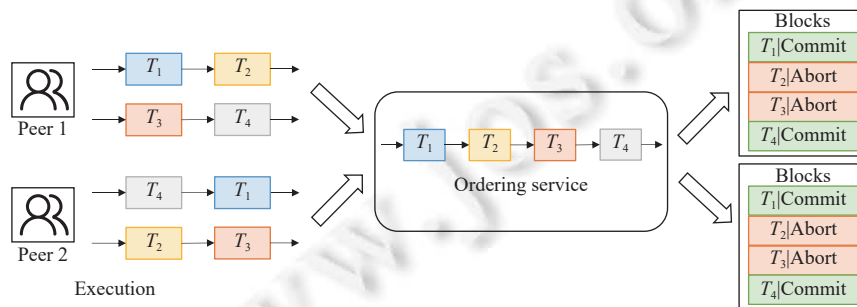
图 7 Fabric 的 OCC 执行流程
