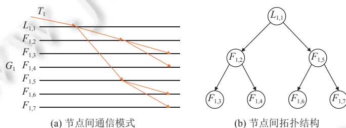
图4 Kauri 在 7 节点时的树形共识流程
