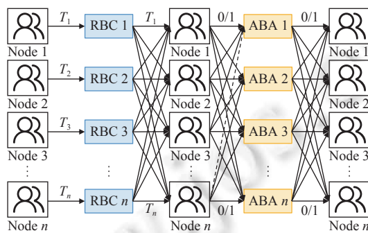
图 6 HB-BFT 的异步共同子集 (ACS) 结构
