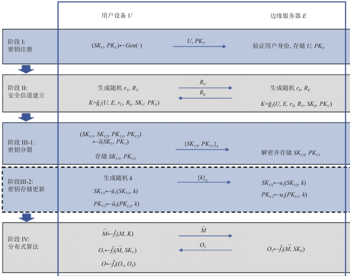
图 2 工作流程
