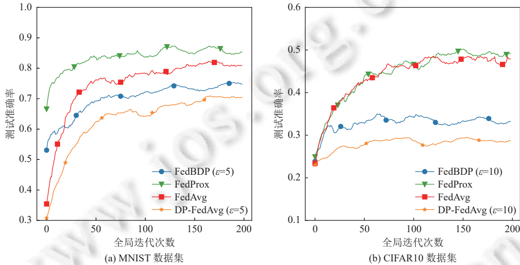
图 6 模型准确率对比
