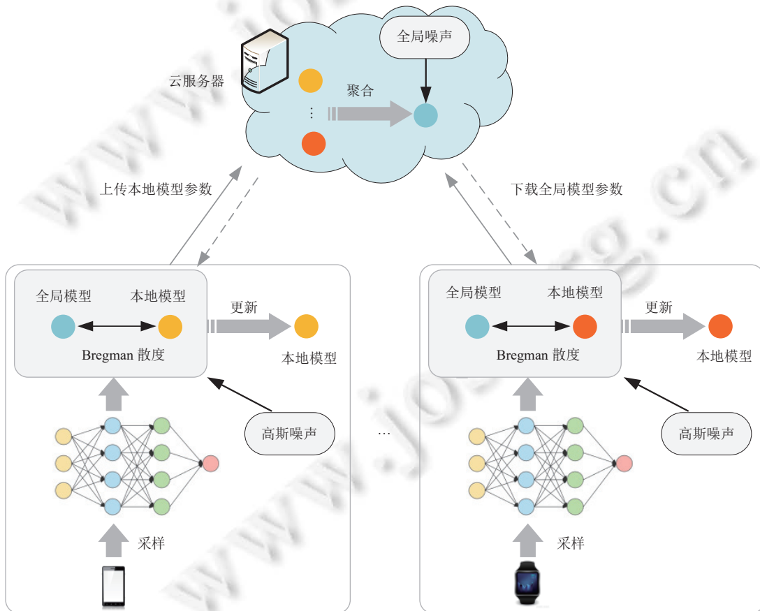
图 1 FedBDP 模型框架
