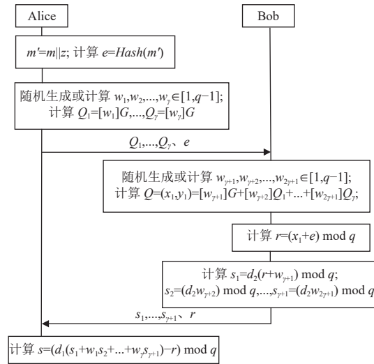
图2 基于乘法密钥拆分的多随机数两方门限计算方案框架
