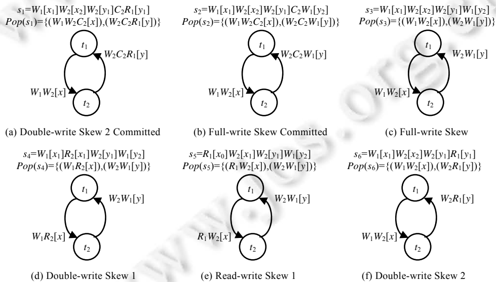
图 11 双元数据异常 PCG 图
