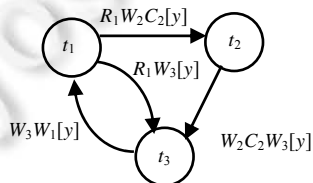
图 1 调度 s 的蕴涵事务状态的冲突图模型
