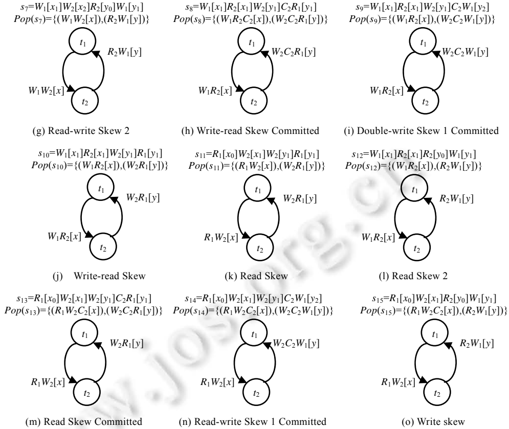
图 11 二元数据异常 PCG 图(续)
