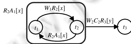
图 5 调度 s 的偏序对图
