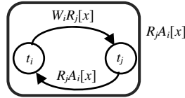
图 2 偏序对 R_jA_i 自身构成偏序环
