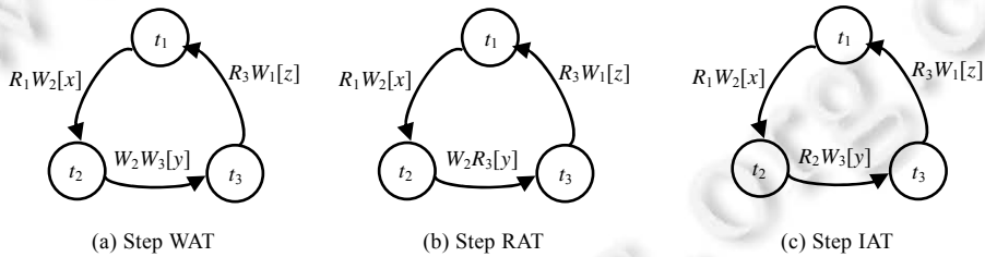
图 12 多元数据异常 PCG 图
