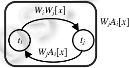
图 4 偏序对 W_jA_i 自身构成偏序环
