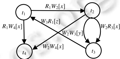
图 6 调度 s_1 的偏序对图
