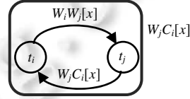
图 3 偏序对 W_jC_i 自身构成偏序环
