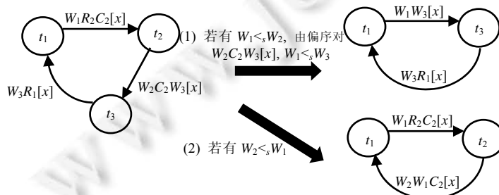
图 7 3 事务单变量偏序环可规约为二事务单变量偏序环
