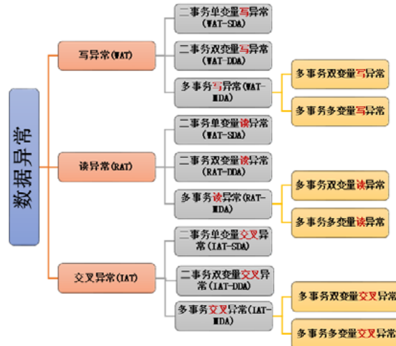
图 9 数据异常类别结构图
