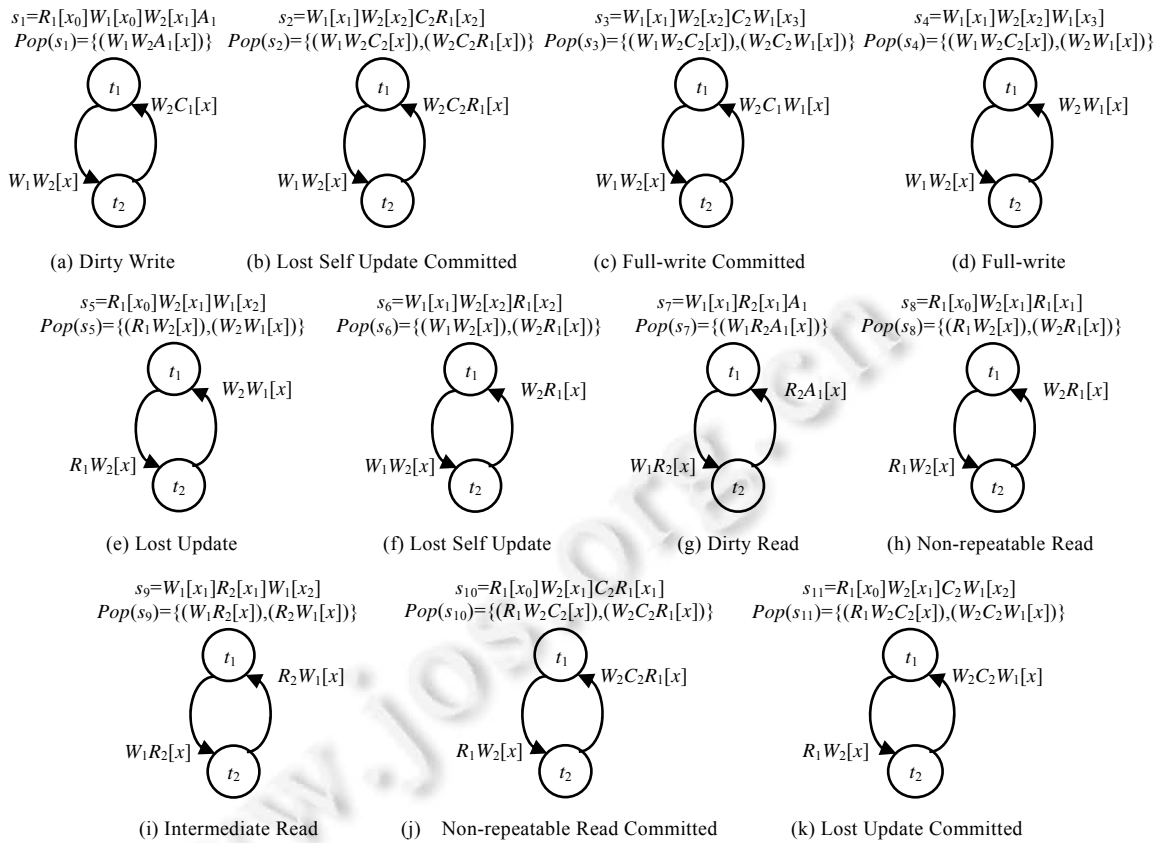
图 10 单元数据异常 PCG 图
