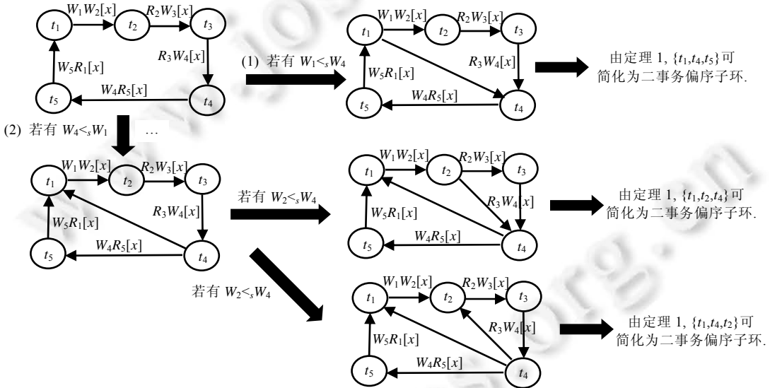
图 8 5 事务单变量偏序环可规约为二事务单变量偏序环
