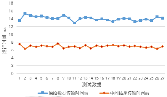
Fig.14 Information transmission time 图 14 信息传输时间
