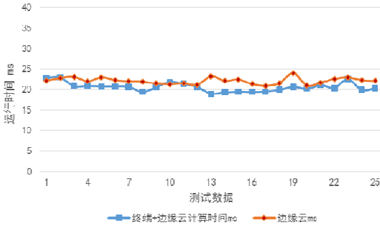
Fig.13 Same calculation task total processing time 图 13 相同计算任务总处理时间
