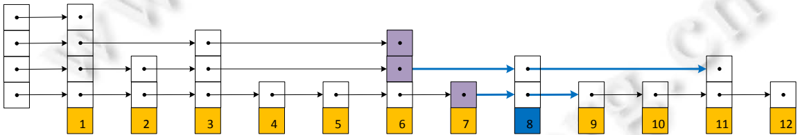
Fig.4 Example of insert node 8 in skip list 图 4 插入结点 8 的示例
