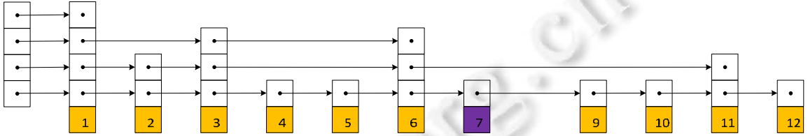
Fig.3 Example of searching node 7 图 3 查找结点 7 的示例
