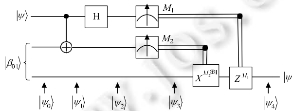
Fig.2 Quantum teleportation for |\beta_{01}\rangle 图 2 关于 |\beta_{01}\rangle 的量子隐形传态
