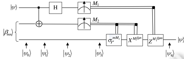
Fig.5 Universal circuit for single-qubit quantum teleportation 图 5 单比特量子隐形传态通用线路
