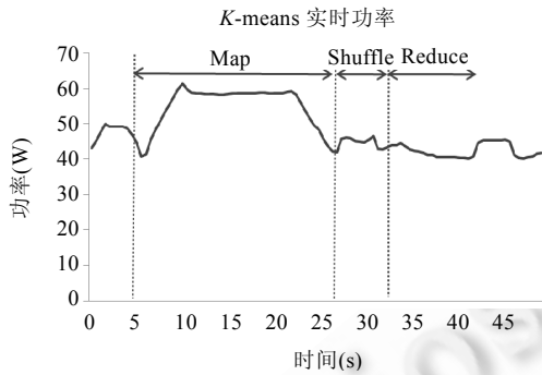
Fig.3 Realtime power (K-means) 图 3 实时功率(K-means)
