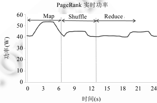
Fig.4 Realtime power (PageRank) 图 4 实时功率(PageRank)
