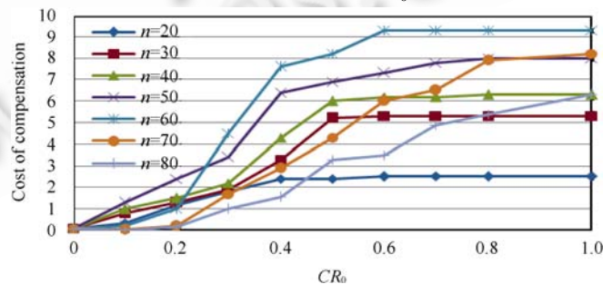
Fig.4 Different CR_0 comparison 图 4 不同风险阈值的对比
