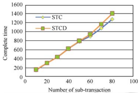
Fig.2 Complete time comparison 图 2 事务完成时间对比
