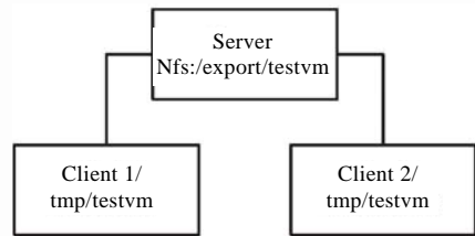
Fig.3 ISR test scenario 图 3 ISR 测试场景
