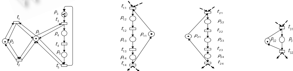
Fig.1 The simple design net system Fig.2 Subnet system 1 Fig.3 Subnet system 2 Fig.4 Subnet system 3 图 1 简单设计网系统 图 2 子网系统 1 图 3 子网系统 2 图 4 子网系统 3
