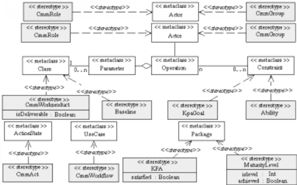
Fig.5 Virtual metamodel of SPM-CMM 图 5 SPM-CMM 的虚元模型
