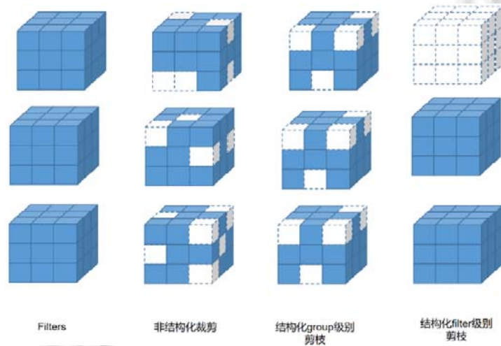
Fig.4 Parameter pruning
