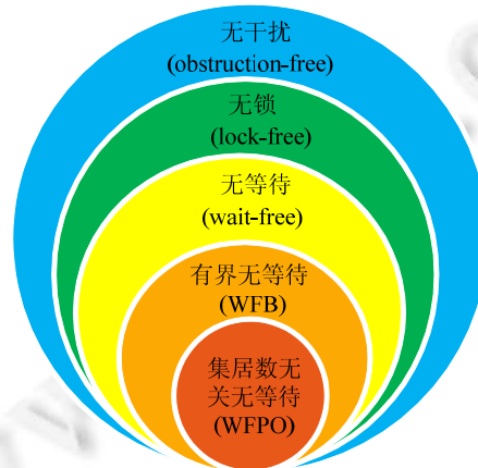
Fig.3 The Venn diagram of non-blocking progress condition 图 3 非阻塞类演进条件的维恩图表示
