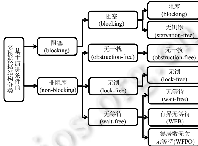
Fig.2 Multi-Core data structure categories based on progress condition 图 2 基于演进条件的多核数据结构分类
