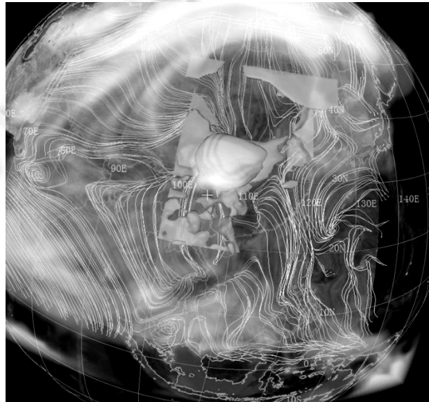
Fig.3 Hybrid rendering result containing streamlines, isosurface and volume rendering 图3 混合绘制结果,图中场景混合了矢量场的流线表达、等值面和体绘制
