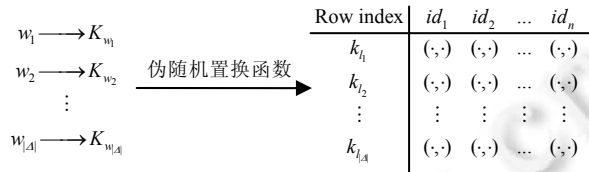
Fig.1 Storage structure of index matrix 图 1 索引矩阵的存储结构
