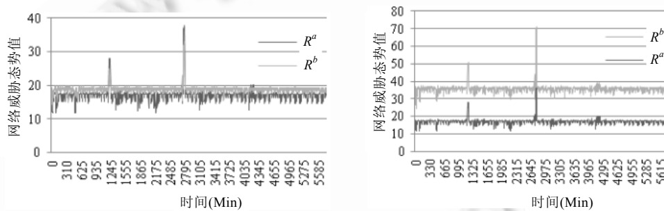
(a) 网络威胁态势值的折线图
