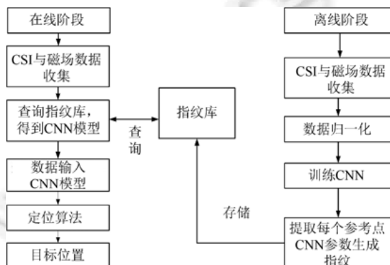
Fig.2 Localization process 图 2 定位过程
