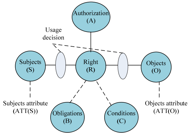
Fig.5 UCON model [25] 图 5 UCON 模型 [25]
