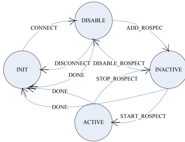
Fig.4 An LTS of IoT reader system 图 4 物联网识读者系统的 LTS
