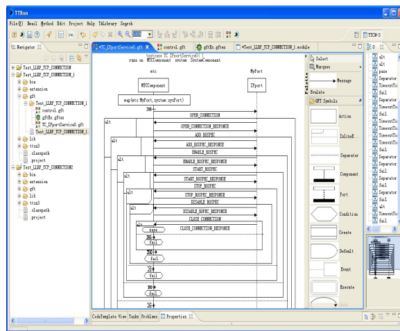
Fig.5 Interface copy of GFT model 图 5 GFT 模型界面
