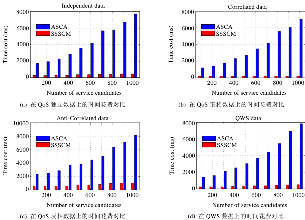
Fig.7 Comparisons on time cost with SSSCM and ASCA 图 7 SSSCM 和 ASCA 的时间花费对比
