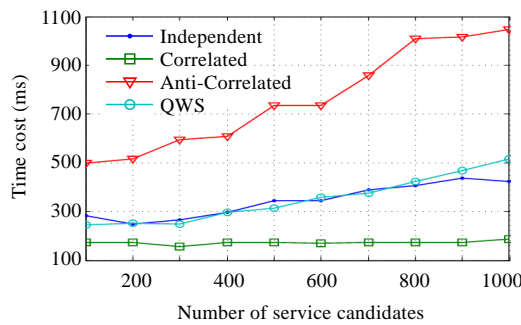
Fig.6 Time cost of SSSCM with respect to four kinds of QoS data 图 6 SSSCM 在 4 种 QoS 数据类型上的时间花费
