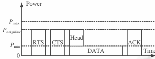
Fig.8 PCSMAC transmit power level 图 8 PCSMAC 发射功率水平
