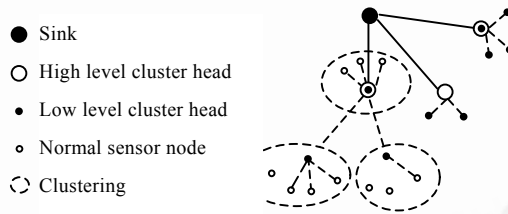
Fig.7 Hierarchical clustering in TEEN protocol 图 7 TEEN 协议中由聚簇构成的层次结构
