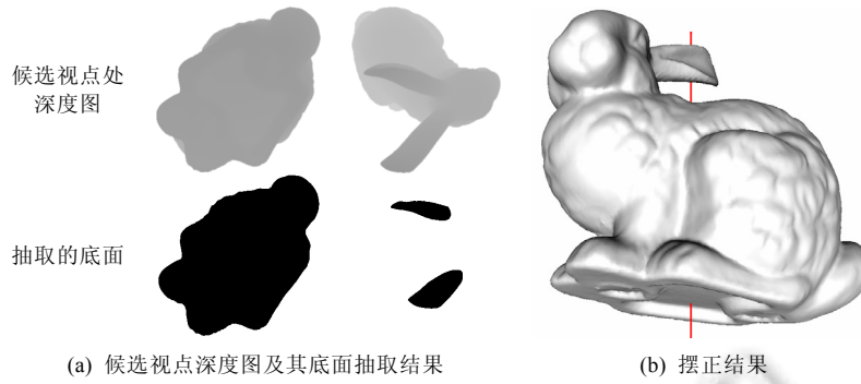
Fig.5 Stability metric 图 5 稳定性准则
