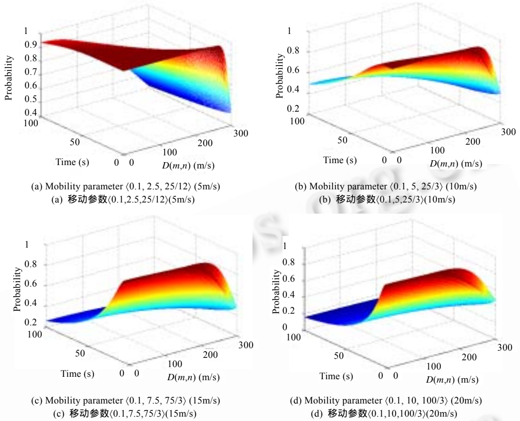
Fig.5 Time- t holding probability P_{m,n}(d,t) of link 图 5 链路的 t -时间维持概率 P_{m,n}(d,t)
