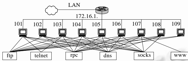
Fig.2 Hierarchical threat evaluation model in HoneyNet network 图 2 HoneyNet 网络系统层次化安全威胁态势评估模型
